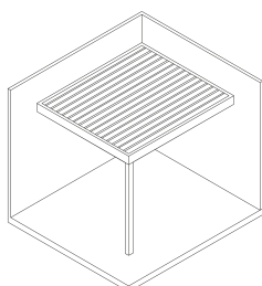
5 Настенное крепление, панели, параллельные стене
