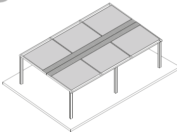
3 Отдельностоящий, шесть модулей
