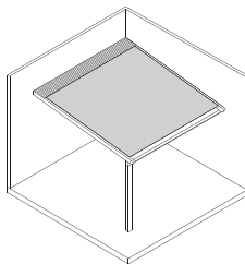
7 Настенное крепление, с двух сторон, одинарный модуль
