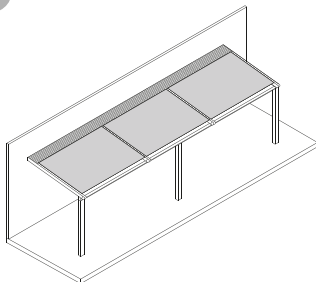
6 Настенное крепление, тройной модуль
